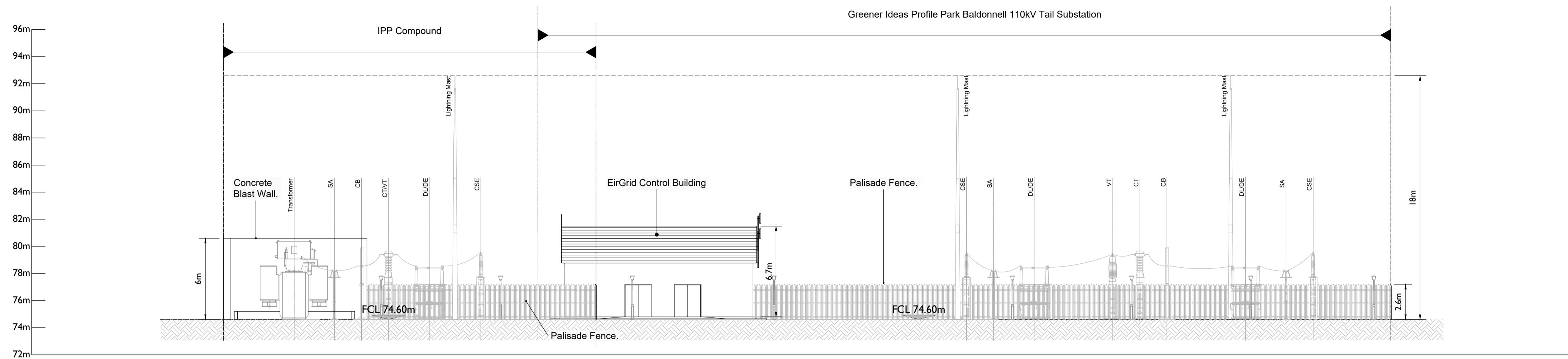
Site Section A-A Scale : 1:200
